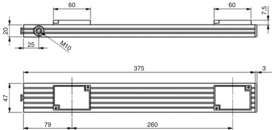
Composant passif F39-TGR-MCL-R-P
