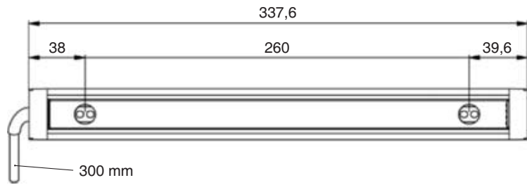
Composant passif F39-TGR-MCL-R-P
