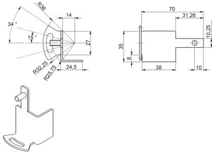
Composant actif F39-TGR-MCL-R-A
