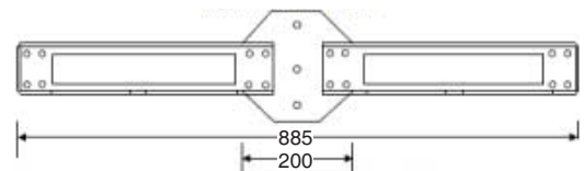
Bras radial d'occultation X- ou T- F39-TGR-AS-MA-MBXT
